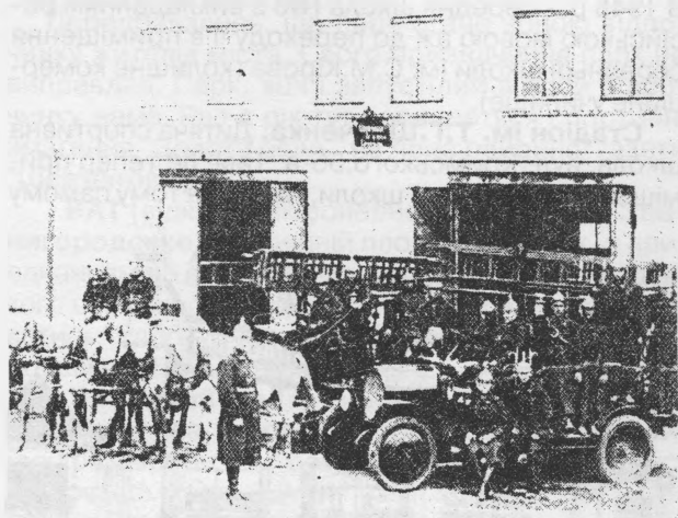
вище: баскі коні, міцні пожежники, здебільшого вусаті, в шаленому русі. Перехожі заздалегідь да-
