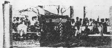
115 років від дня народження МОВЧАНА Василя Архиповича (І. (І4) І. 1903, с.Неморок — 2.VI.1964, Київ) — іхтіолог-рибовод.
